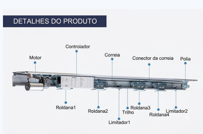
Motor, controlador e roldanas reforçadas
