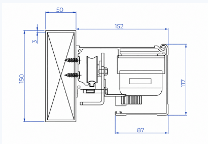
Projeto dimensional preciso
